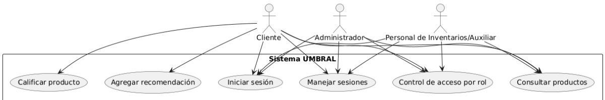
Diagrama general de casos de uso - Sistema UMBRAL
