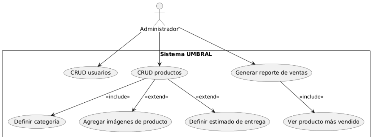
Diagrama general de casos de uso - Sistema UMBRAL
